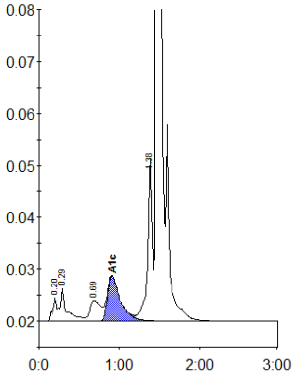
Peak table - ID: 10337253
